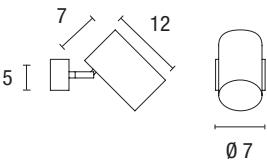
Wall 1x Spot
